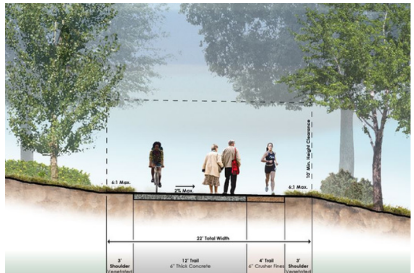
Sección transversal del sendero regional Denver Parks and Recreation
